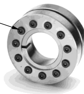
Spannschraube Locking screw Vite trasmettitrice di tensione
