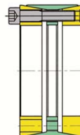
DOBIKON 1015 + Rheinbraun- Spannsatz
